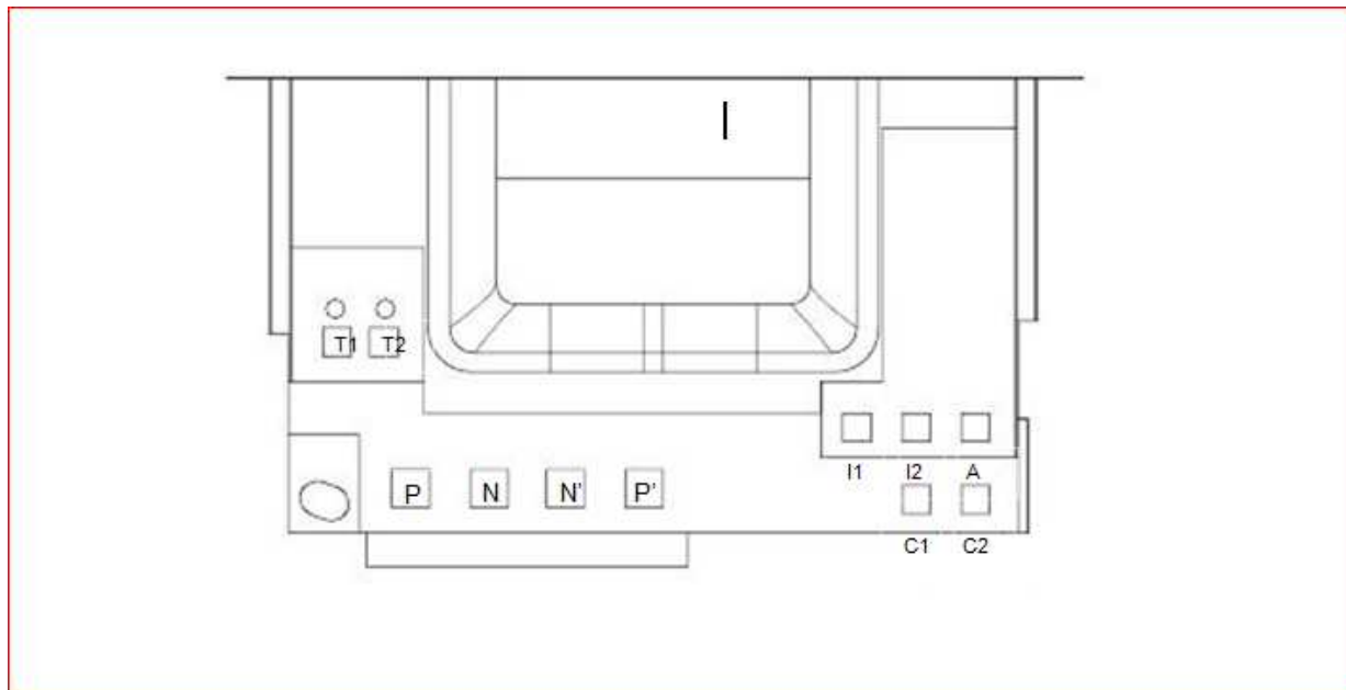
Schéma des borniers du compteur monophasé :
